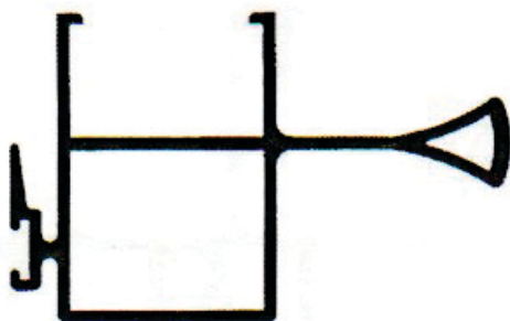
251 M Parante central con tirador hoja DVH Peso 0.808 kg/m
