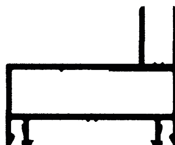
201 M Jamba de marco corrediza Peso 0.750 kg/m
