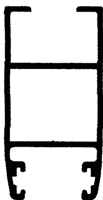
203 M Parante lateral corredizo Peso 0.700 kg/m
