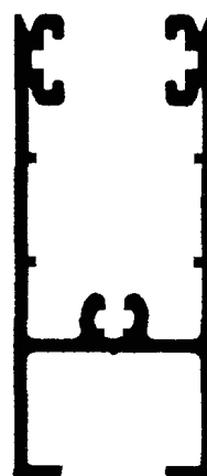
204 M Zócalo y cabezal corrediza Peso 0.720 kg/m
