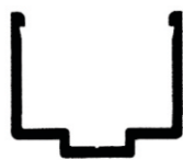
166 M Adaptador para DVH hojas corredizas Peso 0.333 kg/m
