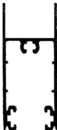
249 M Zócalo y cabezal de hoja para DVH ventana y puerta corrediza Peso 0.658 kg/m
