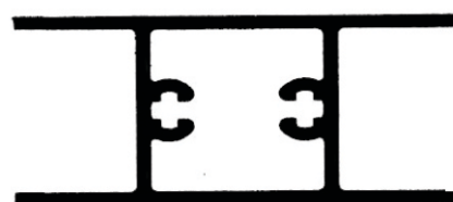
253 M Travesaño de hoja DVH Peso 0.658 kg/m
