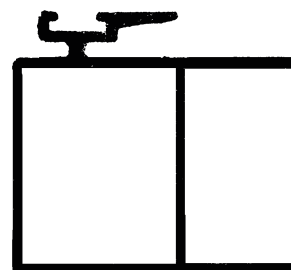
250 M Parante central de hoja para DVH ventana y puerta corrediza Peso 0.653 kg/m
