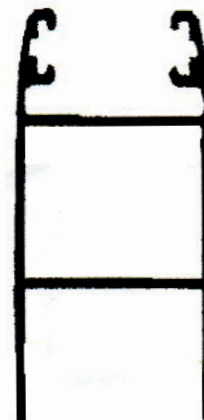
248 M Parante lateral de hoja para DVH ventana y puerta corrediza Peso 0.650 kg/m
