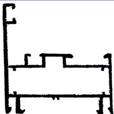
210 M Marco ventana de abrir con cámara compensadora Peso 0.825 kg/m
