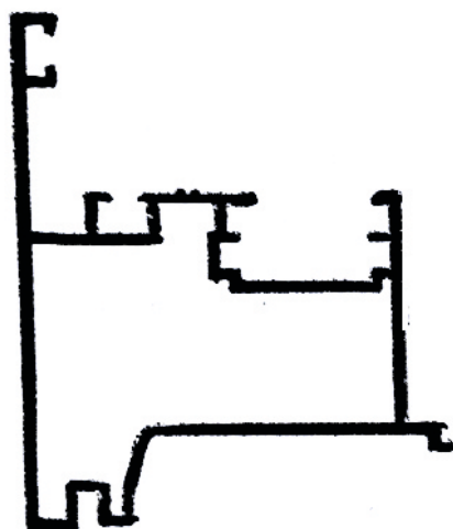
223 M Encuentro central ventana de abrir 2 hojas con cámara compensadora Peso 1.033 kg/m
